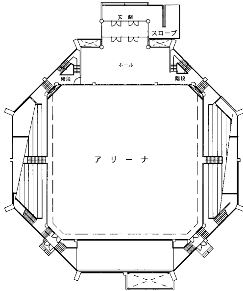
1階 平面図
