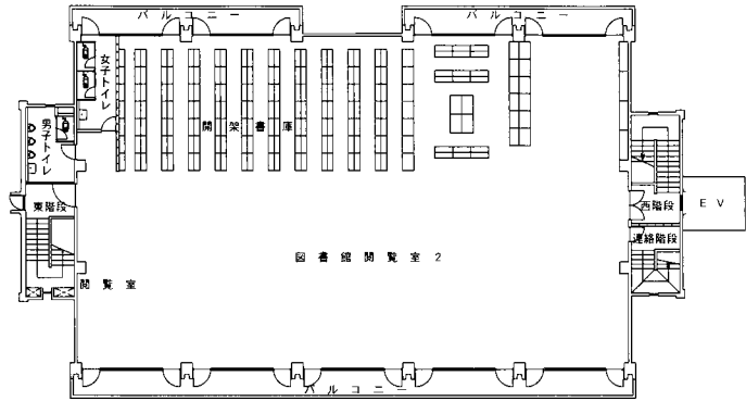
3階 平面図
