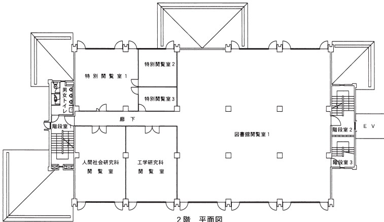
2階 平面図
