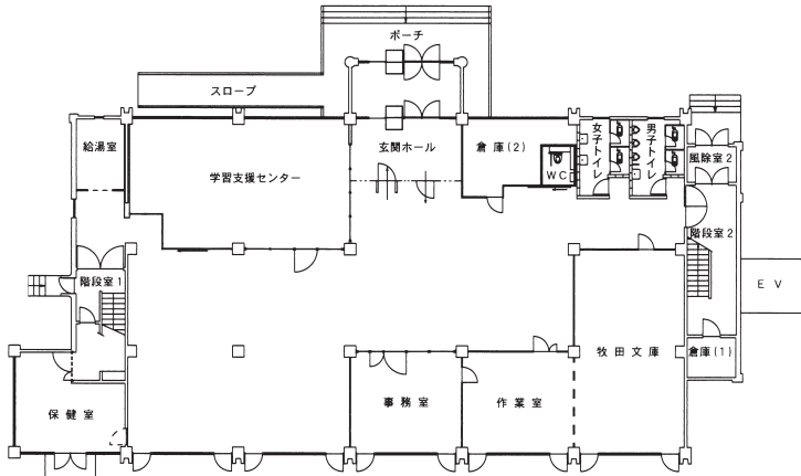
1階 平面図
