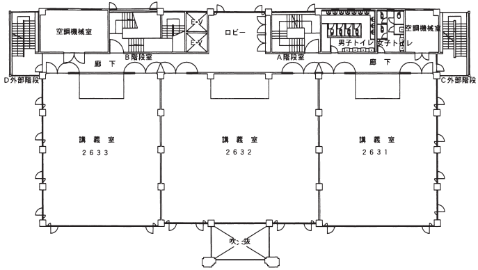
3階 平面図
