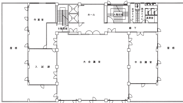
4階 平面図
