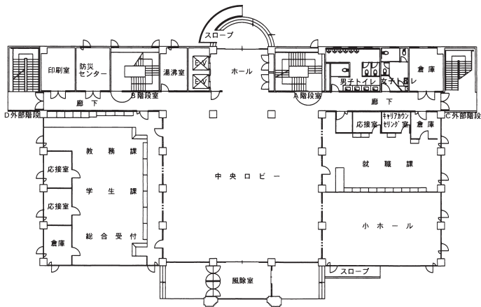
1階 平面図
