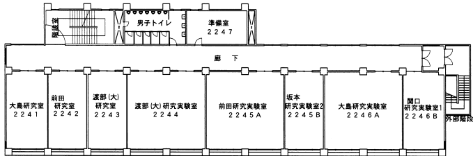
4階 平面図
