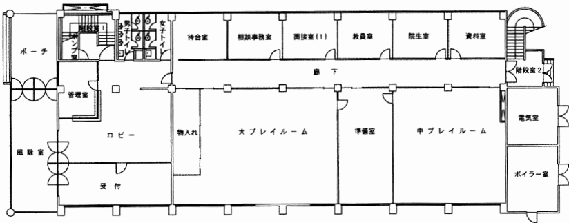
1階 平面図
