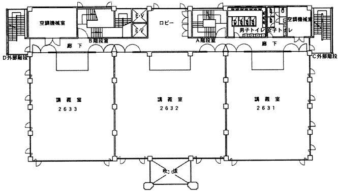
3階 平面図
