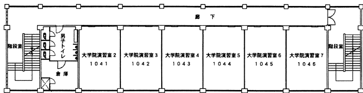
4階 平面図
