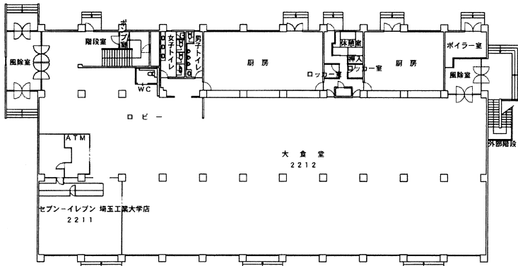
1階 平面図
