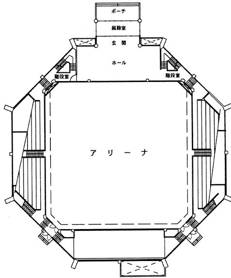
1階 平面図
