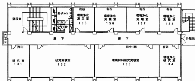
3階 平面図
