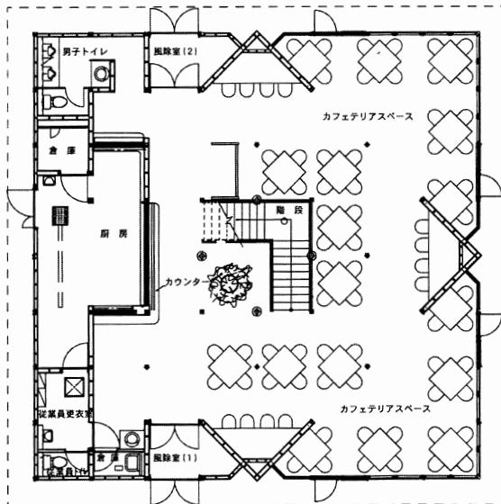
1階 平面図
