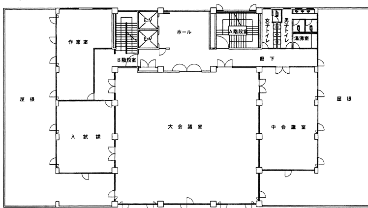
4階 平面図
