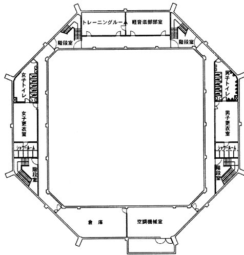
地階 平面図
