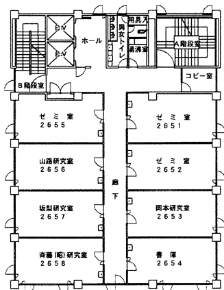
5階 平面図
