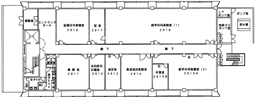
1階 平面図
