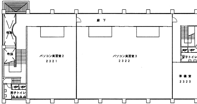
2階 平面図
