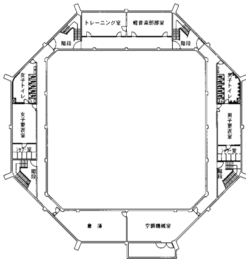
地階 平面図
