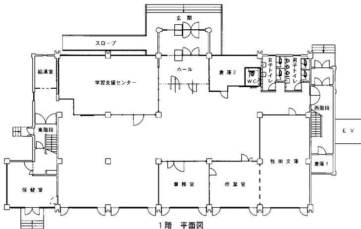
1階 平面図
