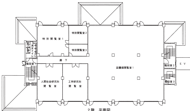
2階 平面図
