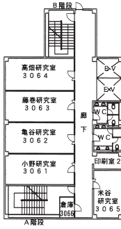
6階 平面図
