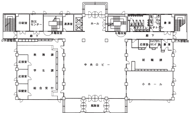
1階 平面図
