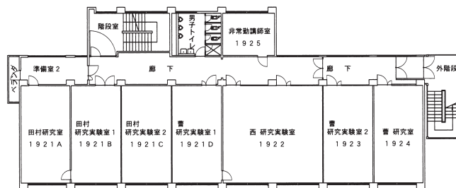
2階 平面図
