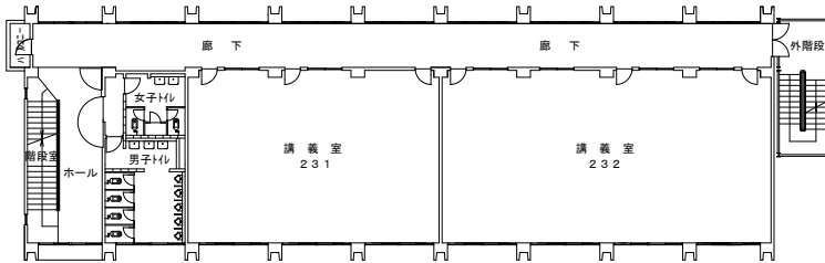
3階 平面図
