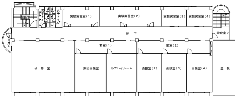
2階 平面図
