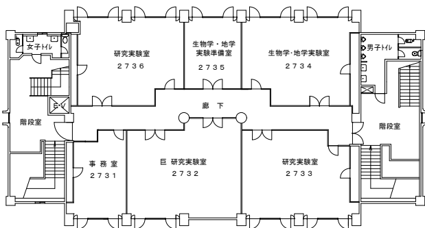
3階 平面図
