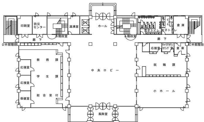
1階 平面図
