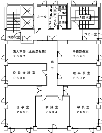
9階 平面図
