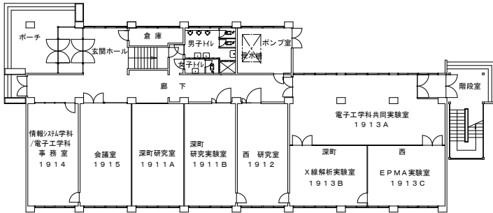
1階 平面図
