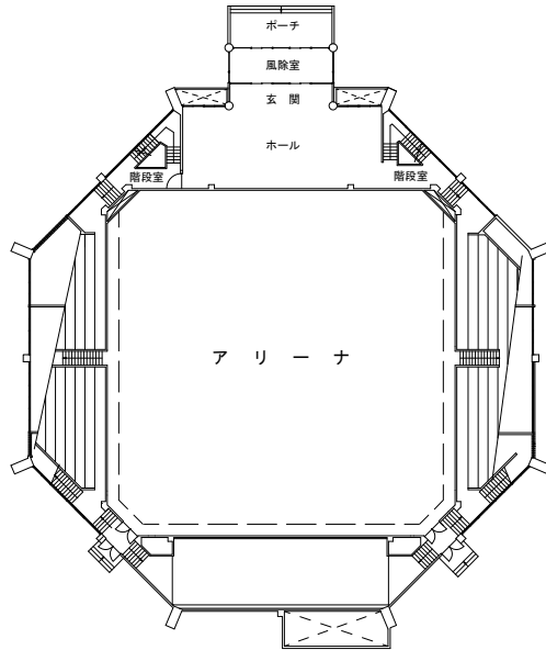
1階 平面図
