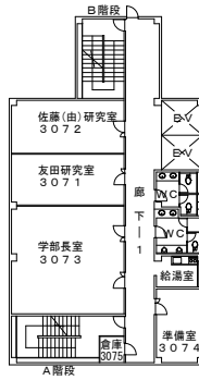
7階 平面図
