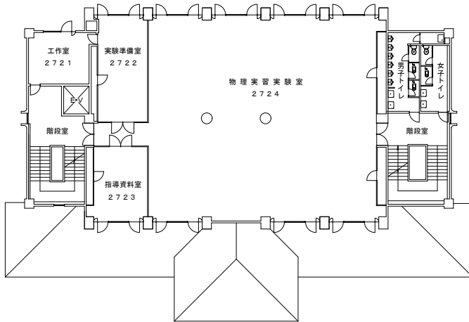
2階 平面図
