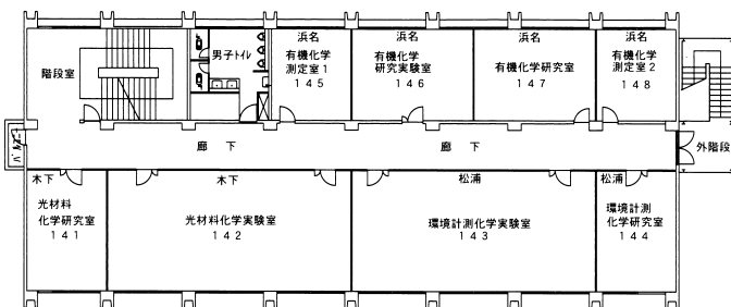
4階 平面図
