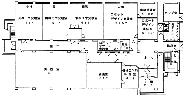
1階 平面図
