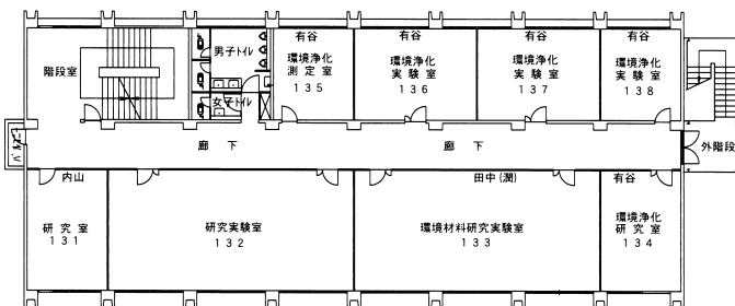
3階 平面図
