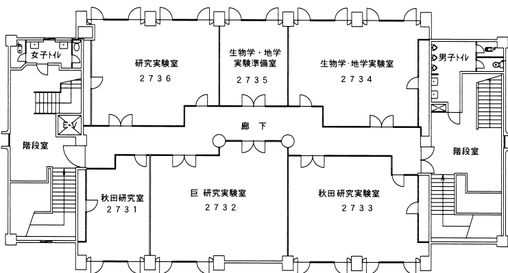
3階 平面図
