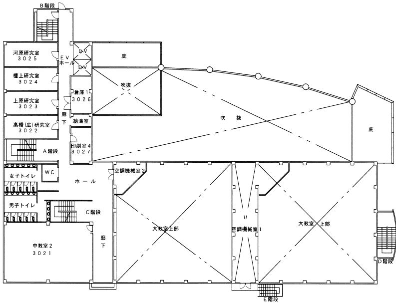
2階 平面図
