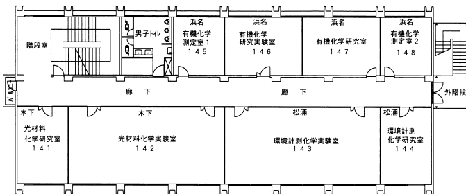
4階 平面図
