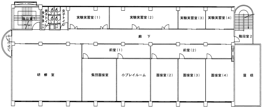
2階 平面図
