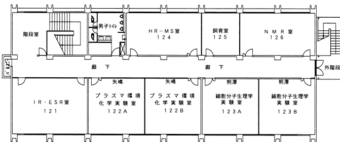
2階 平面図
