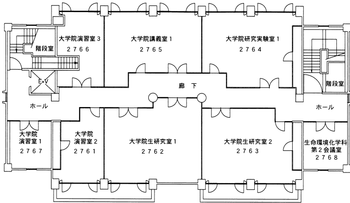
6階 平面図
