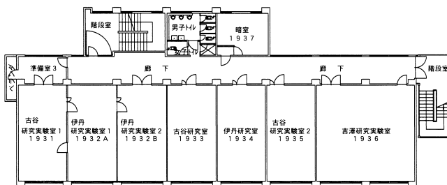
3階 平面図
