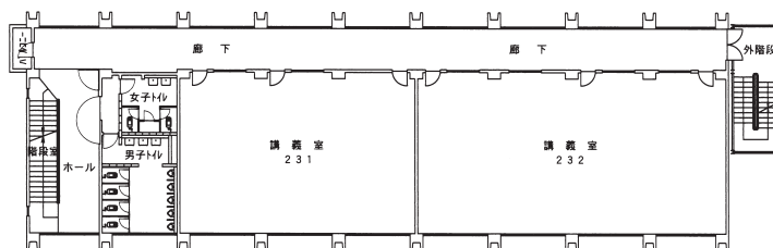
3階 平面図
