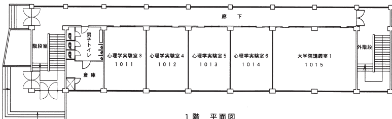
1階 平面図
