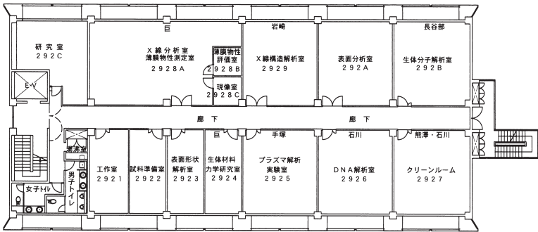
2階 平面図
